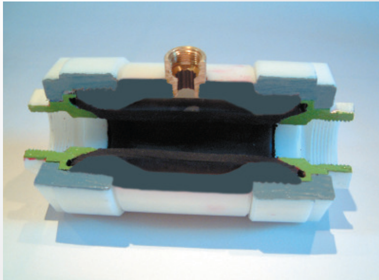
Quetschventil im Querschnitt
